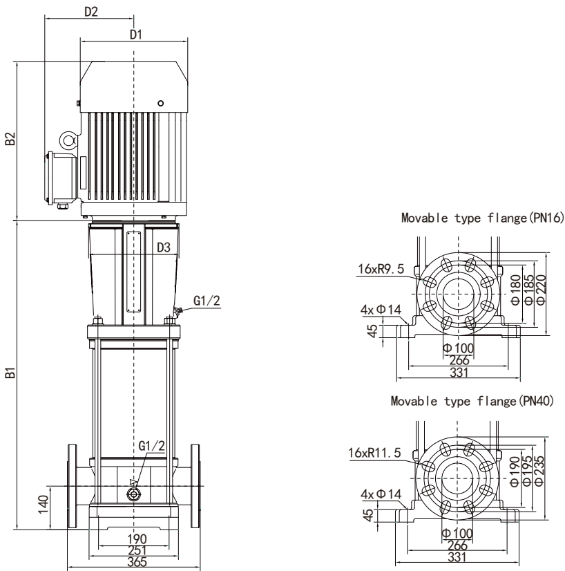
DIN 标准适用: PN10~PN40/DN100
