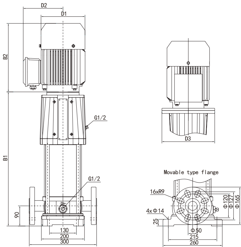
DIN 标准适用: PN10~PN40/DN50
