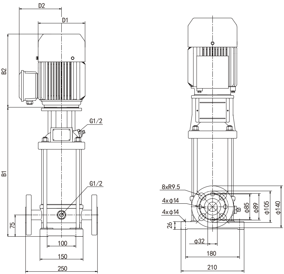
DIN 标准适用: PN10~PN40/DN32
