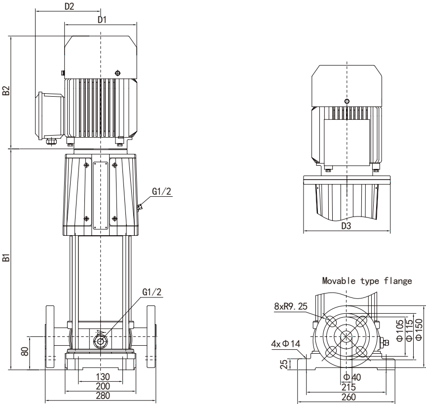
DIN 标准适用: PN10~PN40/DN40
