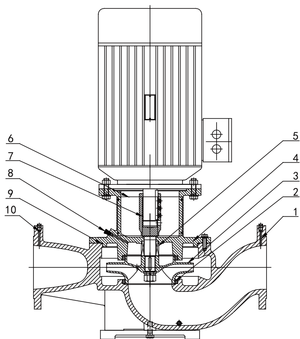
Structure Chart ( DP32~DP150 )
