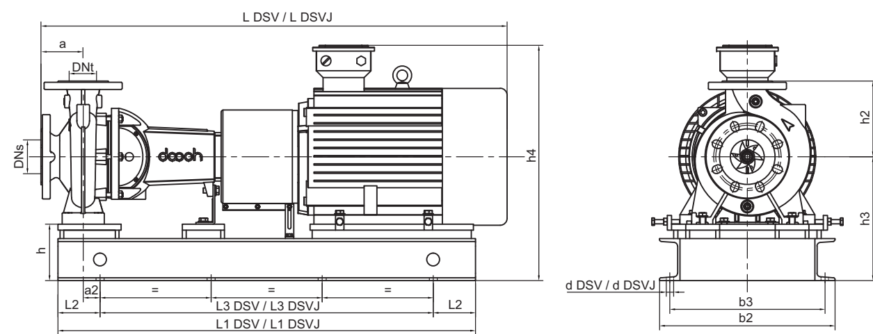
DSV (J) 类型C
