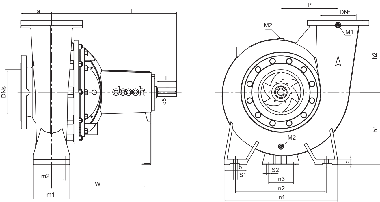
泵头尺寸（切向出口）： DSV (J)
