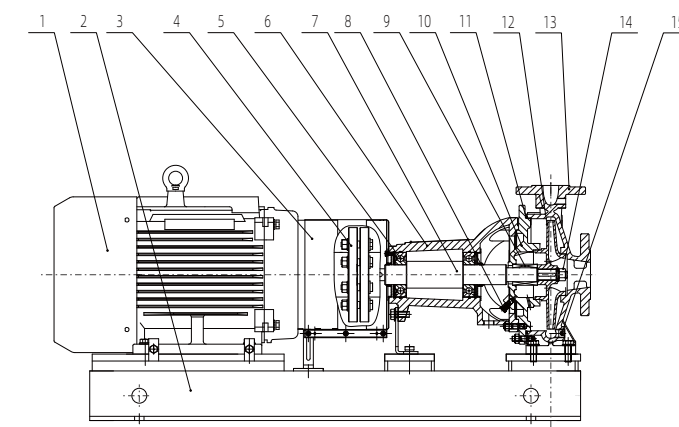
1. DSV结构示意图及主要零件及材料:
