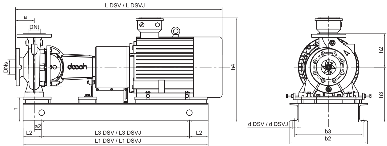
DSV (J) 类型A
