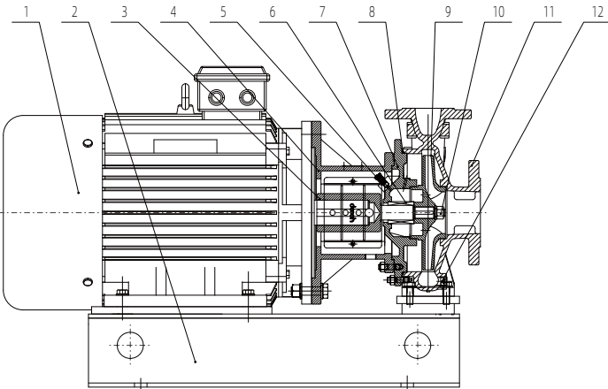
3. DSVG结构示意图及主要零件及材料:
