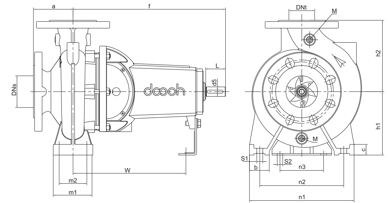
泵头尺寸（中心线出口）： DSV (J)
