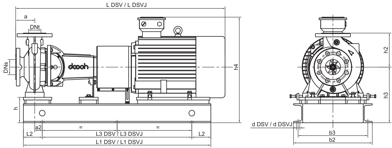
DSV (J) 类型B
